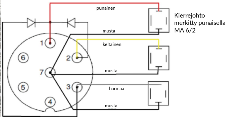
KHK200 "Original" Snowstar zoom, aura taittuu virrattomana
