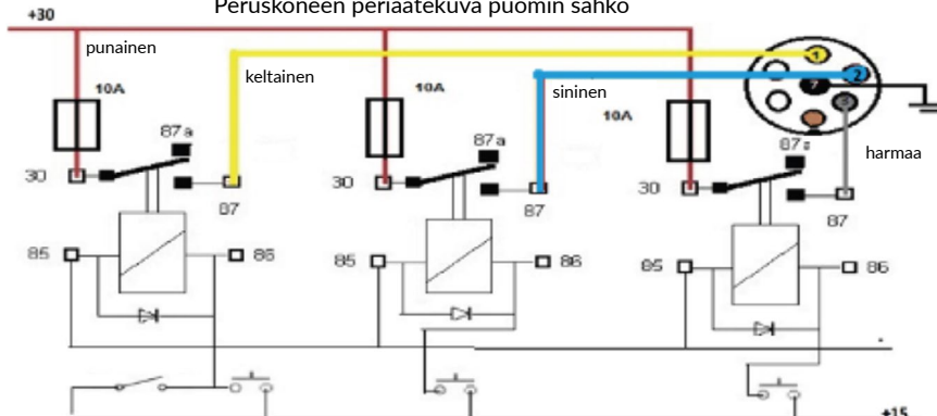
Peruskoneen periaatekuva puomin sähkö
