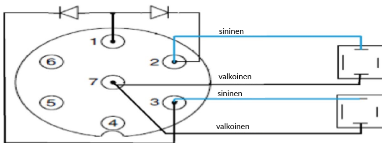
KHK207 "Snowstar" zoom versio 2 kahdella kelalla, virrattoman aura taittuu
