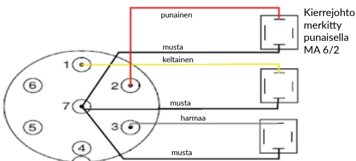
KHK208 "Arcon Pro", aura leviää virrattomana
