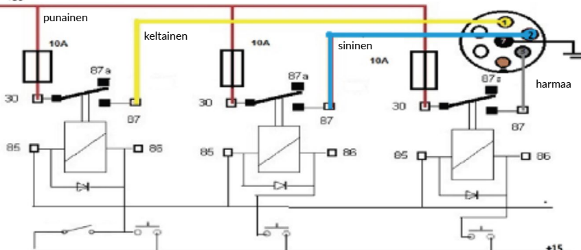
Peruskoneen periaatekuva puomin sähkö
