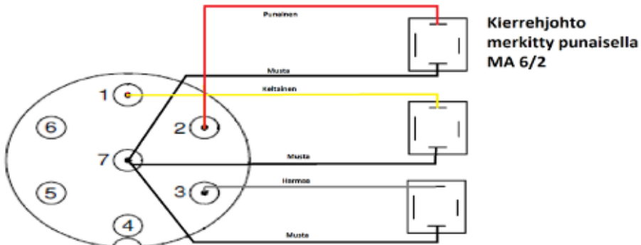
KHK208 "Arcon Pro", Aura leviää virrattomana
