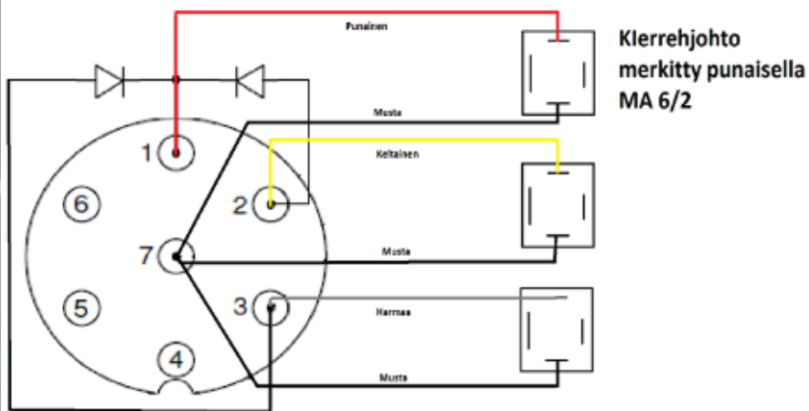
KHK200 "original" Snowstar Zoom, Aura taittuu virrattomana
