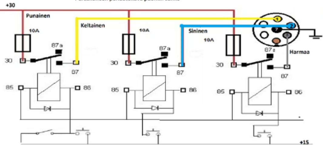
Peruskoneen periaatekuva puomin sähkö
